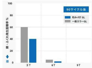
耐食性 180度曲げ加工部の耐食性試験結果
